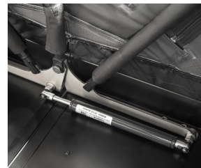
Vérins à gaz pour une ouverture et une fermeture faciles / Gasdruckfedern zum leichten Auf- und Zuklappen
